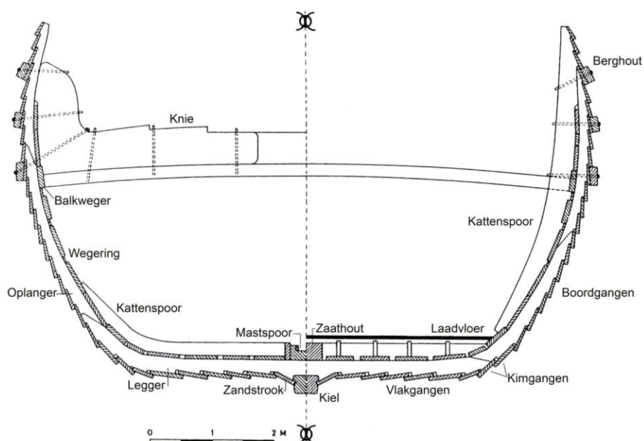
Afb. Doorsnede van een overnaads gebouwd schip (tekening. R. Oosting, RCE)
