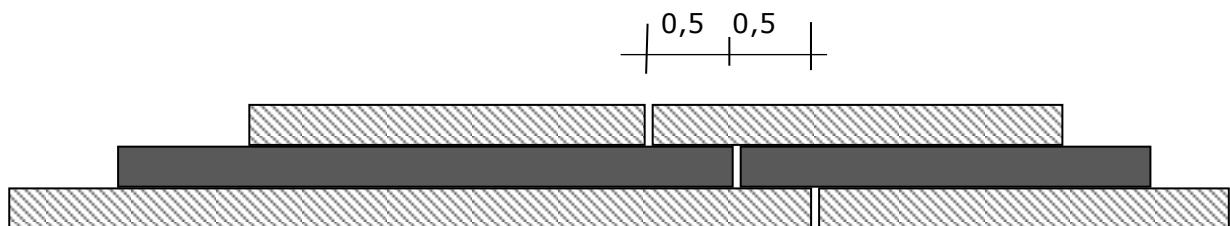
Figuur 1: Verspringende naden bij meerdere asfaltlagen
