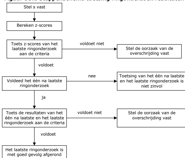
Figuur B5.1 Stappenschema toetsing ringonderzoek resultaten
