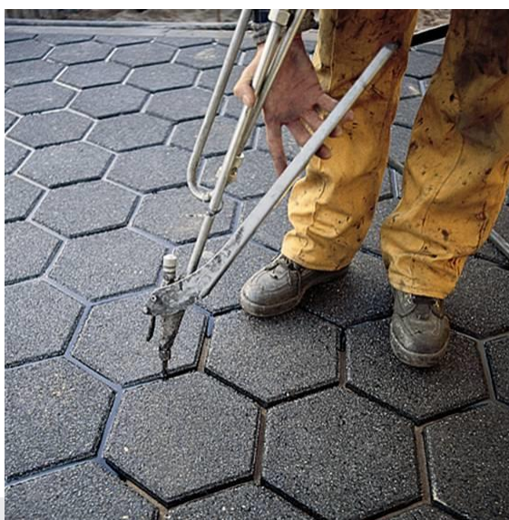
Foto: aanbrengen van voegvulmassa.
