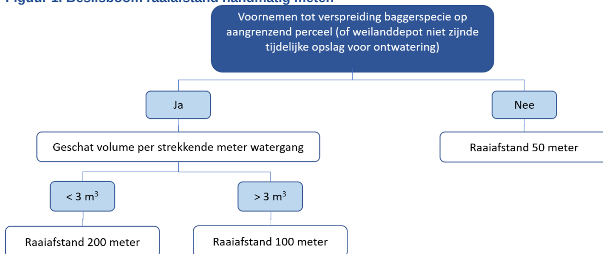
Figuur 1. Beslisboom raaiafstand handmatig meten
